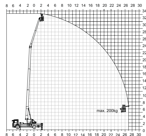
Bühnenbetrieb* (HA 2/200) · Klappspitze 1x ausgezogen
